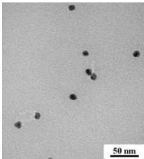
Obr. Sférické paládiové nanočástice v transmisním elektronovém mikroskopu
